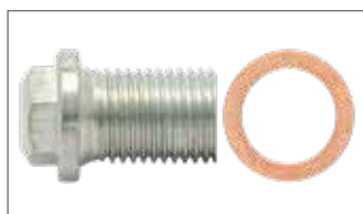
Ölablassschraube mit Dichtring (Stahl, Zinklamellenbeschichtet DP)
